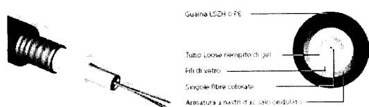
Cavo in fibra ottica armato da esterno
