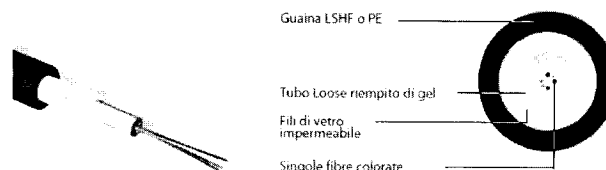
Cavo in fibra ottica di tipo loose
